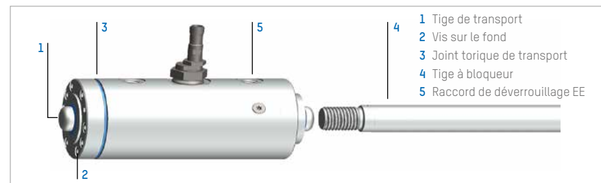
Illustration 12 : Installation du bloqueur de tige Ratio-Clamp® avec tige de transport
