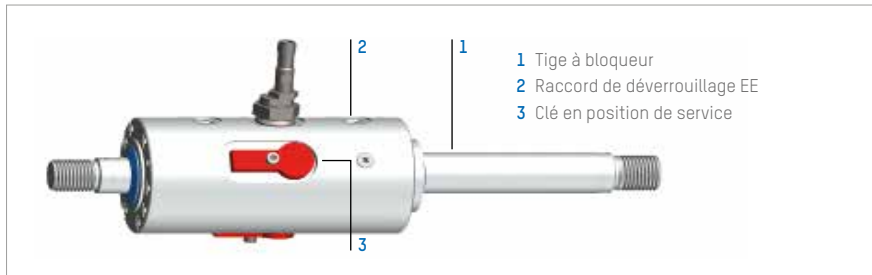
Illustration 14 : Installation du bloqueur de tige Ratio-Clamp® avec clé en position de service
