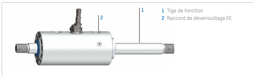
Illustration 11 : Installation du bloqueur de tige Ratio-Clamp® avec tige de fonction
