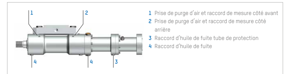
Illustration 5 : Prises de purge d'air et raccords de mesure du système de joints du vérin Servofloat® ou Servoseal®
