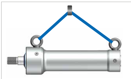
Illustration 2 : Utilisation d'œillets de transport
