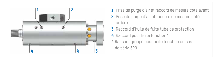
Illustration 6 : Prises de purge d'air et raccords de mesure du système de joints du vérin Servofloat®
