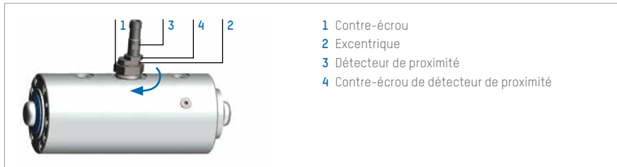
Illustration 16 : Régler le détecteur de proximité sur verrouillé
