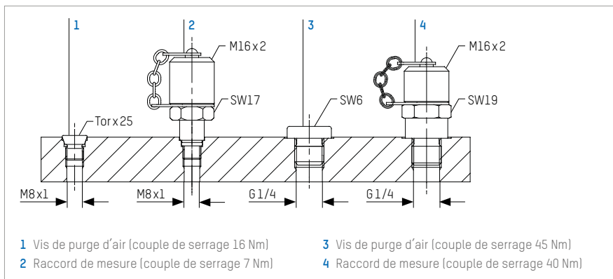
Illustration 8: Vis de purge couples de serrage
