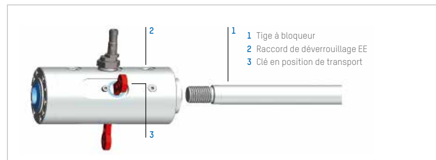
Illustration 13 : Installation du bloqueur de tige Ratio-Clamp® avec clé en position de transport
