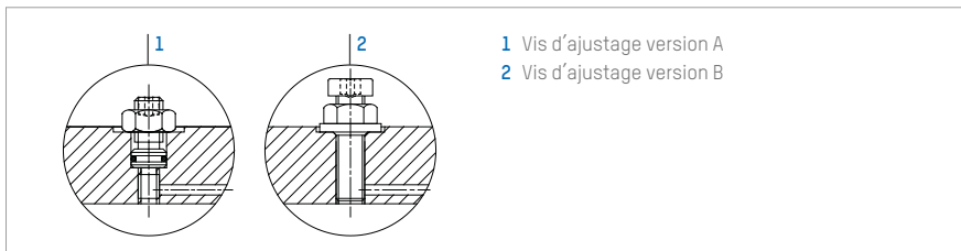
Illustration 10 : Versions de vis d'ajustage amortissement de fin de course
